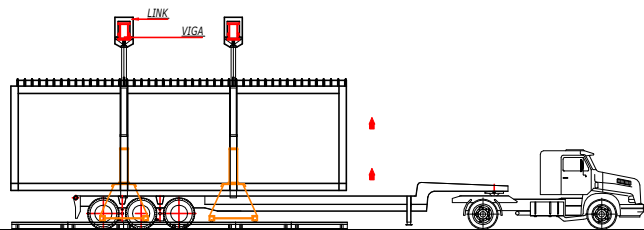
2ª FASE - IÇAMENTO DO CONTAINER E POSICIONAMENTO DA CARRETA.
