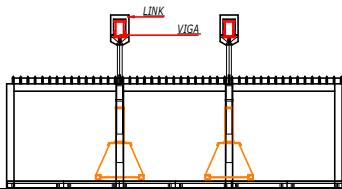
1ª FASE - POSIÇÃO INICIAL DO CONTAINER E PÓRTICO POSICIONADO.
